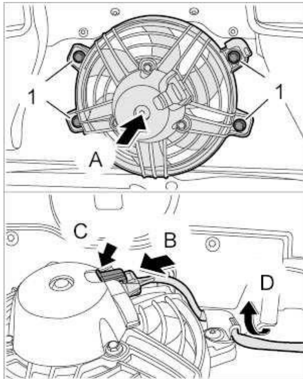
Securing fan motor on rear lid
