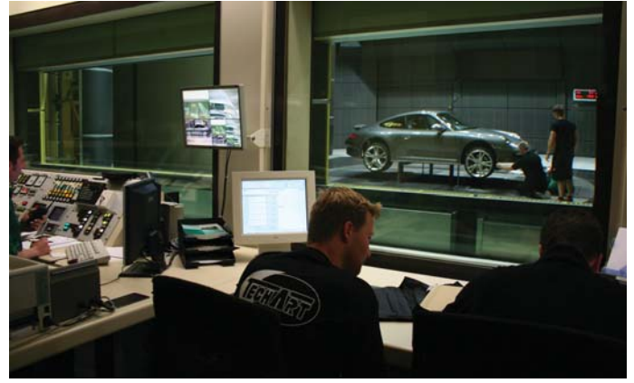
Erprobung der aerodynamischen Komponenten im Windkanal Wind tunnel testing of the aerodynamic components
