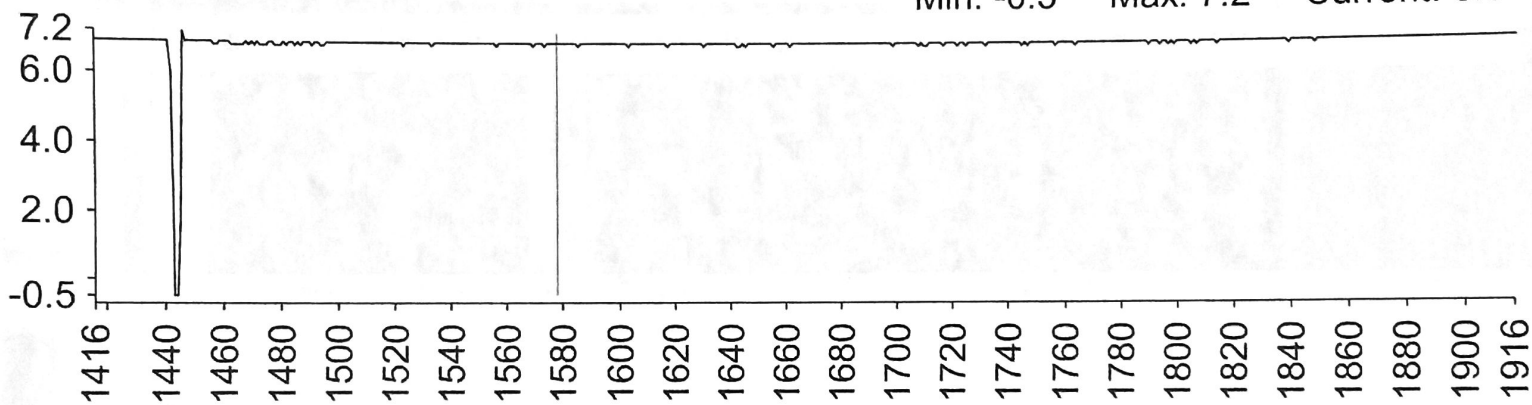
Shift Rod Position, Gears 1 - 3(mm)
